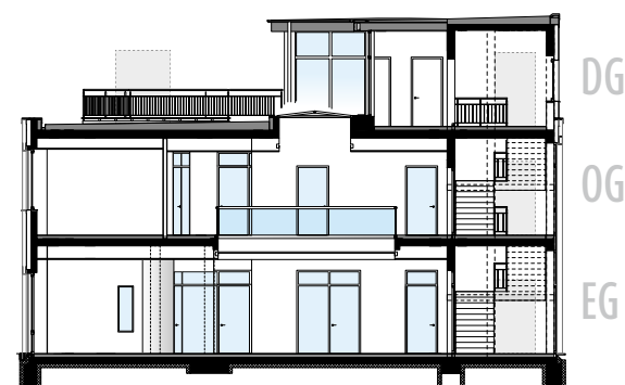
GEBÄUDESNITT
